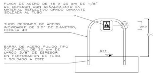
ALZADO
